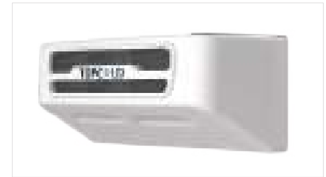
Condensador Dimensiones 1580×715×690(L×W×H/mm)
